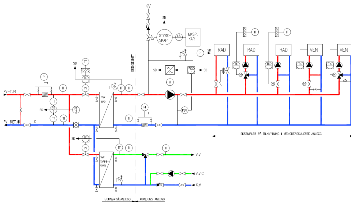
Figur 3. Eksempel på Kundesentral med oppvarming og tappevann
