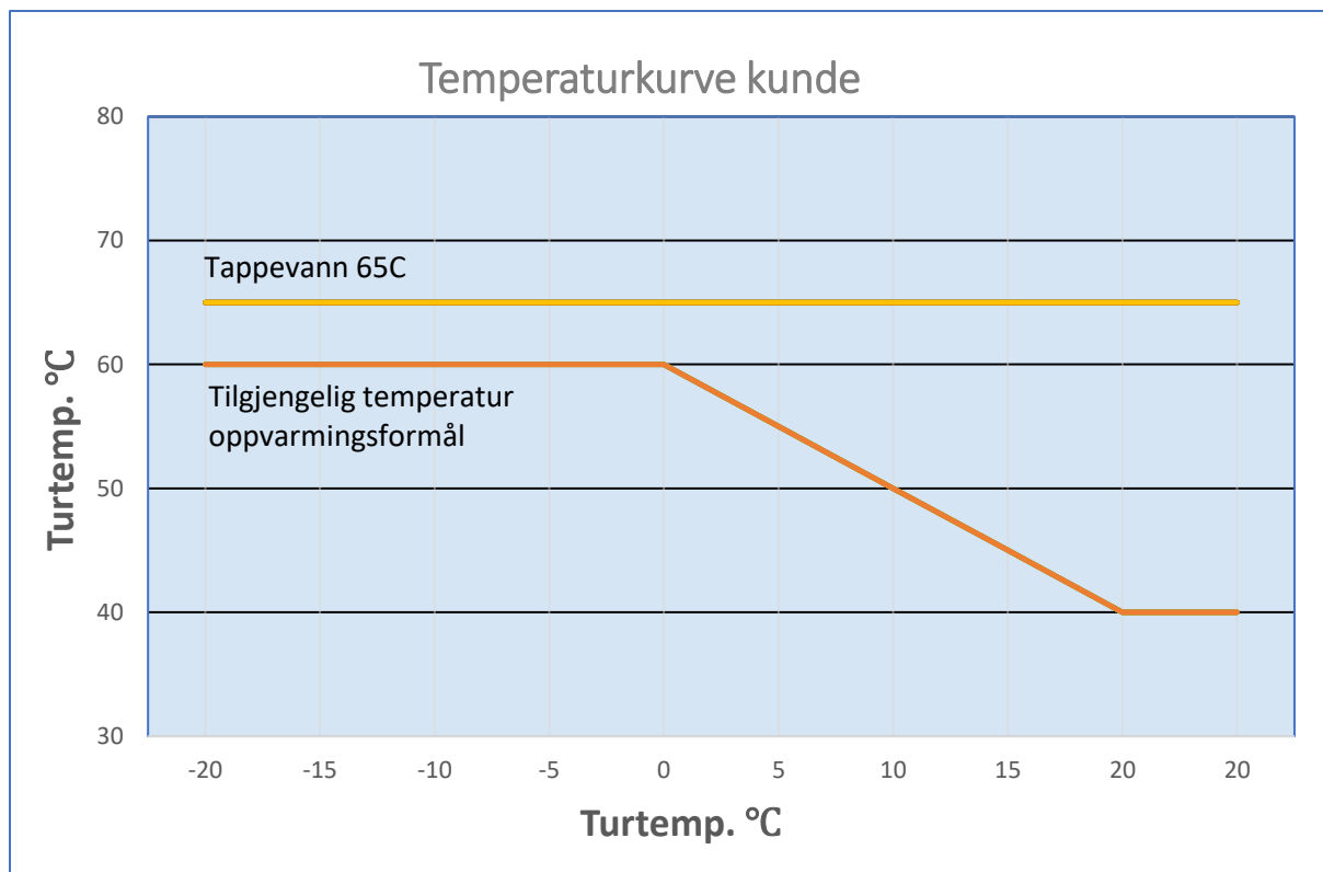
Figur 2. Eksempel på utekompensert varmekurve
